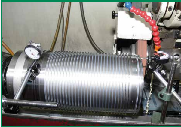
Außenrundscheifen einer Kühlhülse mit eingeschrumpftem 20 KW Stator Outside round grinding of a cooling sleeve with a 20 kW stator, shrunk into position.
